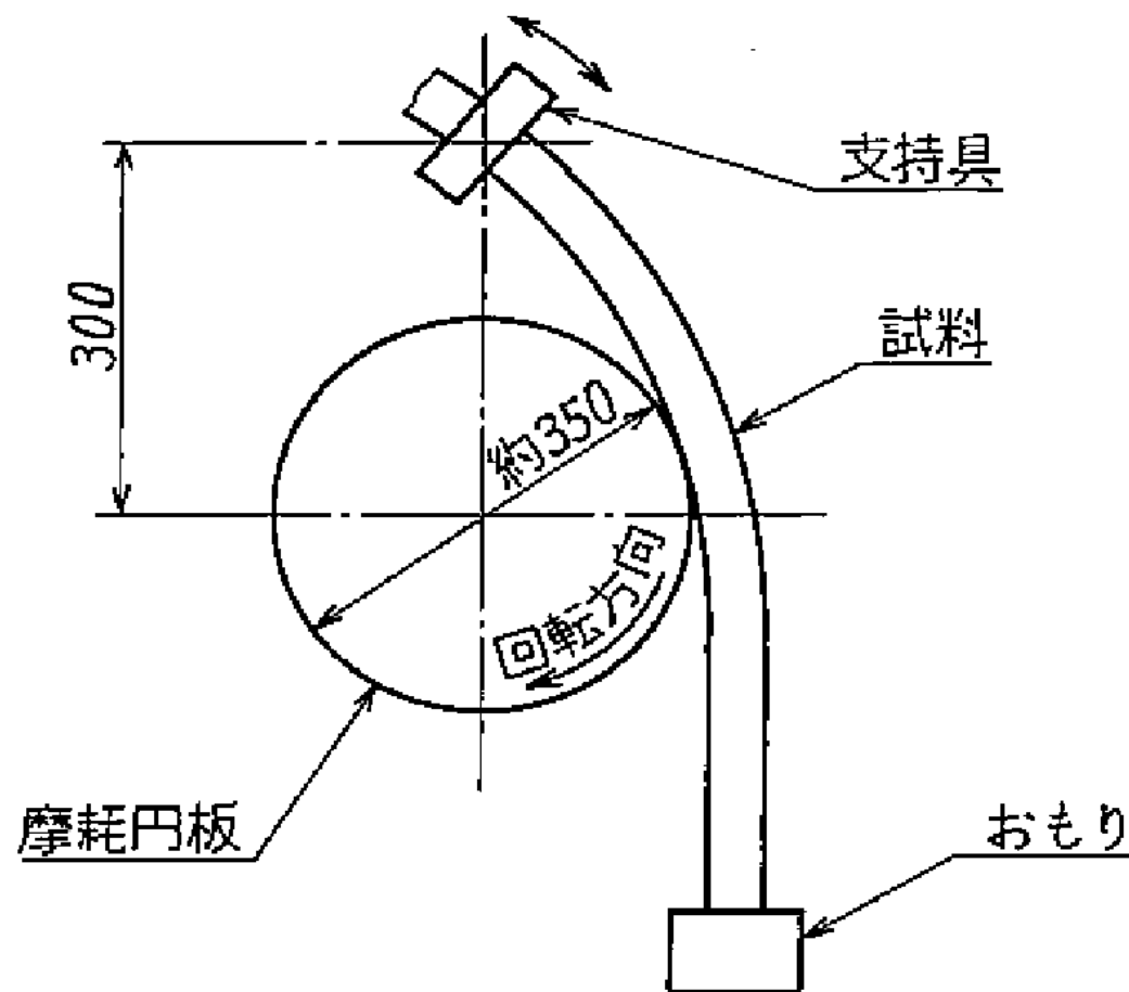
図22 摩耗試験装置
