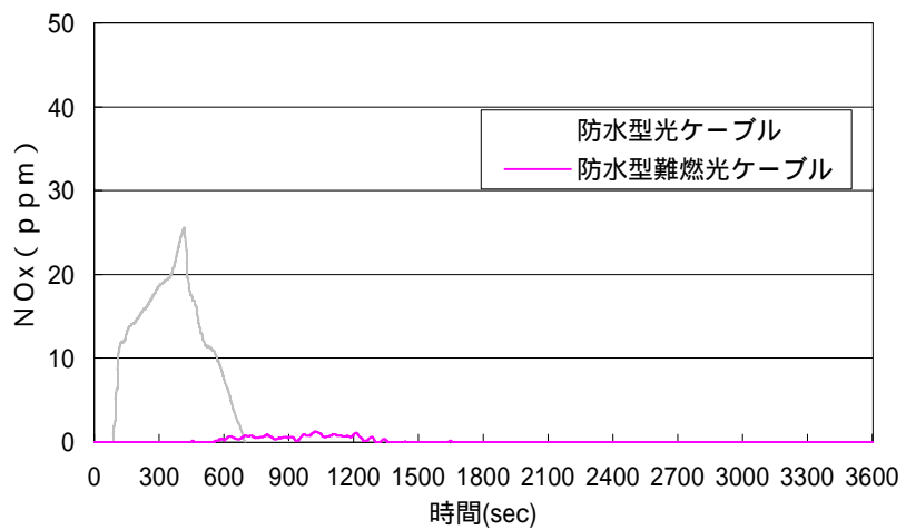
図2.(3)-20 防水型光ケーブルと防水型難燃光ケーブルのNOx発生量 ( 輻射熱量50kW/m 2 )
