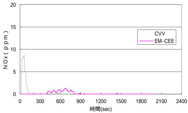
図2.(3)-19 CVVとEM-CEEのNOx発生量 ( 輻射熱量50kW/m 2 )
