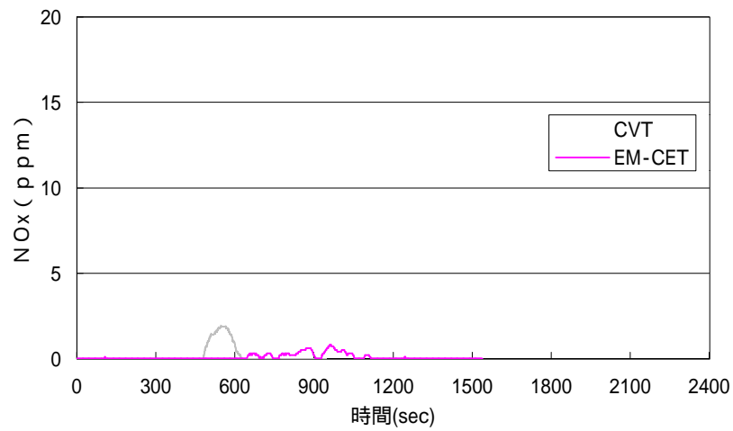
図2.(3)-18 CVTとEM-CETのNOx発生量 ( 輻射熱量50kW/m 2 )
