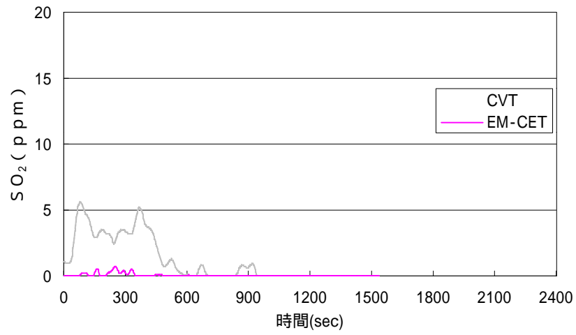
図2.(3)-15 CVTとEM-CETのSO 2 発生量 (輻射熱量50kW/m 2 )
