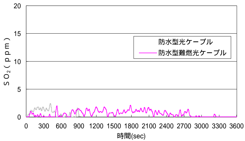
図2.(3)-17 防水型光ケーブルと防水型難燃光ケーブルのSO 2 発生量 (輻射熱量50kW/m 2 )
