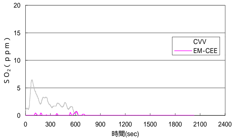
図2.(3)-16 CVVとEM-CEEのSO 2 発生量 (輻射熱量50kW/m 2 )
