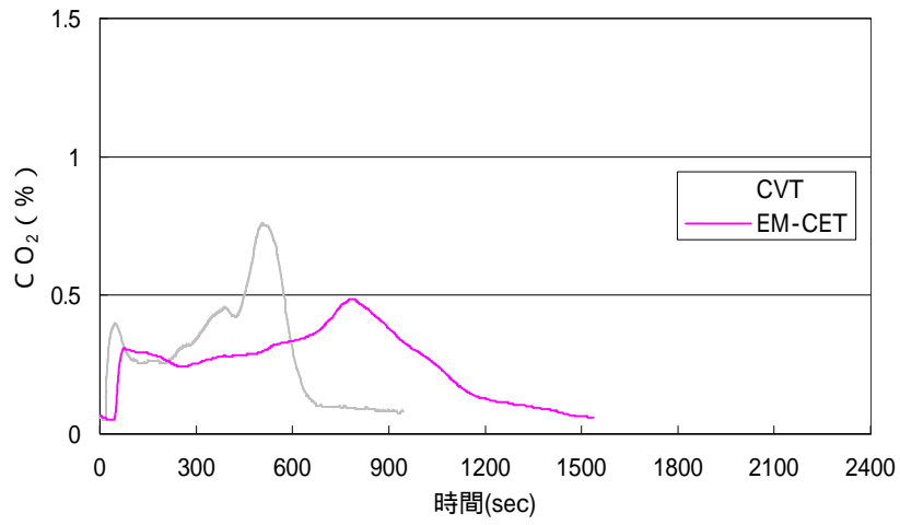
図2.(3)-9 CVTとEM-CETのCO 2 発生量 (輻射熱量50kW/m 2 )
