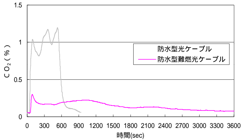
図2.(3)-11 防水型光ケーブルと防水型難燃光ケーブルのCO 2 発生量 (輻射熱量50kW/m 2 )
