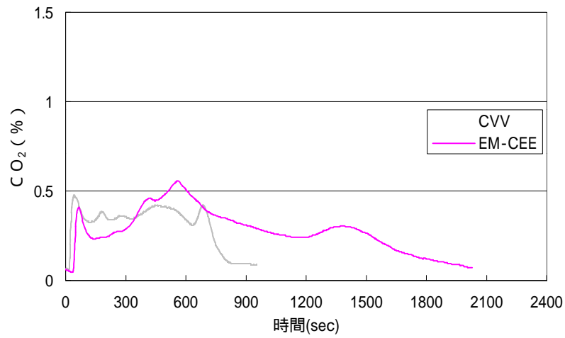
図2.(3)-10 CVVとEM-CEEのCO 2 発生量 (輻射熱量50kW/m 2 )
